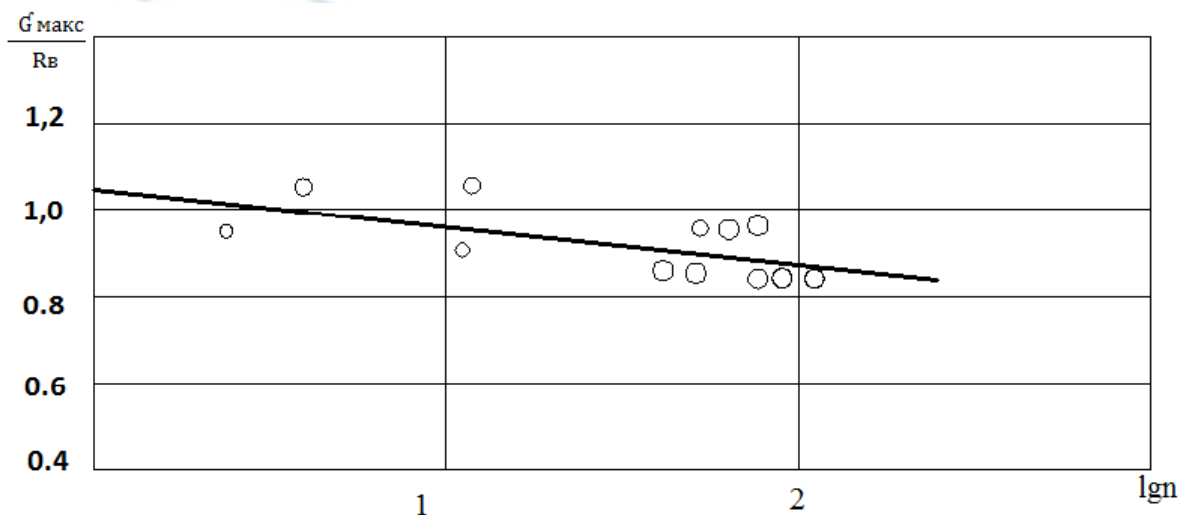
Рис. 1. Результаты испытаний неавтоклавногазозолобетона (III серия) при малоцикловых динамических нагрузках. Критерии оценки достоверности полученных результатов.
