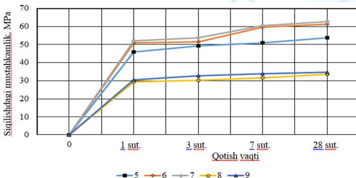
1-rasm. Barxan qumli issiq-nam ishlovi berilgan YuMBning vaqt bo'yicha mustahkamligining o'zgarishi. Tarkiblarning tartib raqami 2 – jadval bo'yicha.
