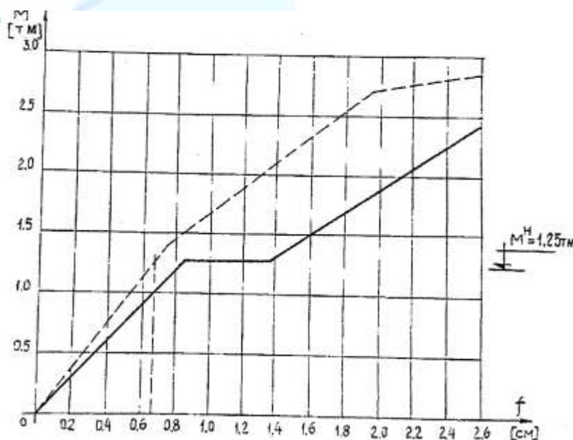
Рис. 1. Прогибы опытных плит в середине пролёта.
