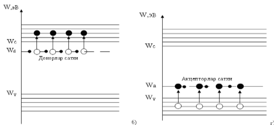
2 – rasm. Kiritmali yarim o'tkazgichlar
