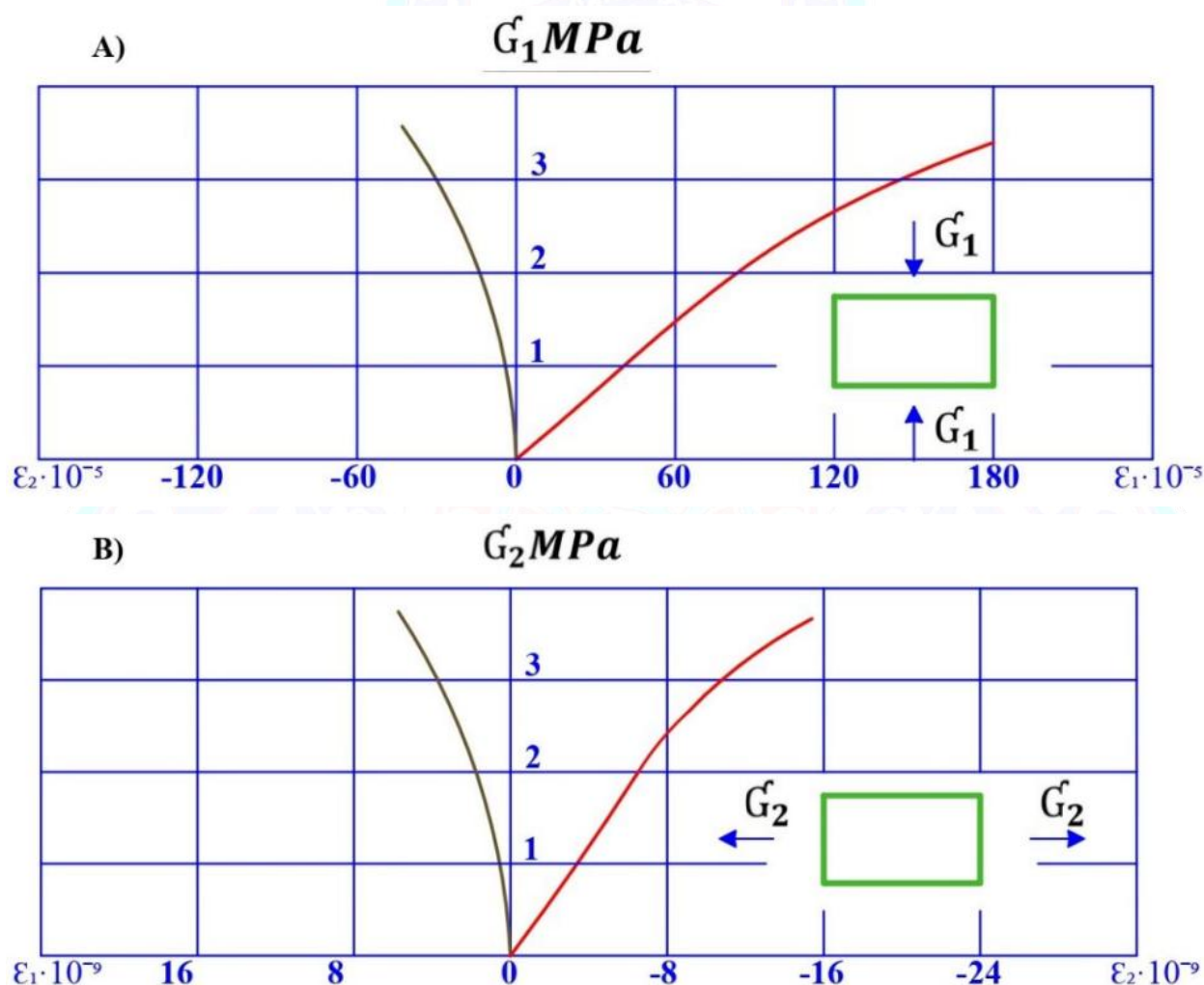
Рис. 1. Характер изменения относительных деформаций неавтоклавного газобетона (на немолотом песке IX серии) при а) центральном сжатии и б) растяжении) (с устранением влияния трения).
